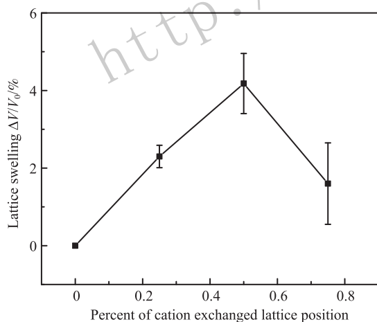
图 4 晶格肿胀程度随交换晶格位置的阳离子比例的变化图
