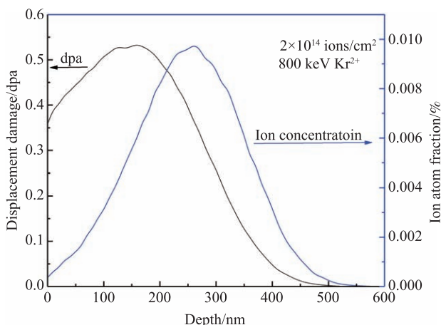
图 1 (在线彩图) 800 keV \text{Kr}^{2+} 在 2.0 \times 10^{14} ions/cm 2 剂量下辐照烧绿石结构 \text{Lu}_2\text{Ti}_2\text{O}_7 的 SRIM 模拟图
