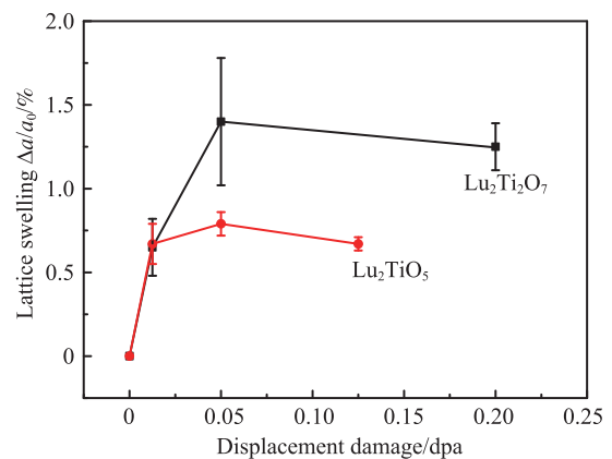
图 3 (在线彩图) 两种材料在 800 keV Kr 2+ 辐照下产生的晶格肿胀随位移损伤的变化
