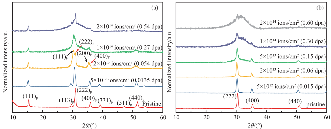
图 2 (在线彩图) Lu 2 Ti 2 O 7 (a)和Lu 2 TiO 5 (b)经 800 keV Kr 2+ 辐照前与辐照后的 GIXRD 谱图
